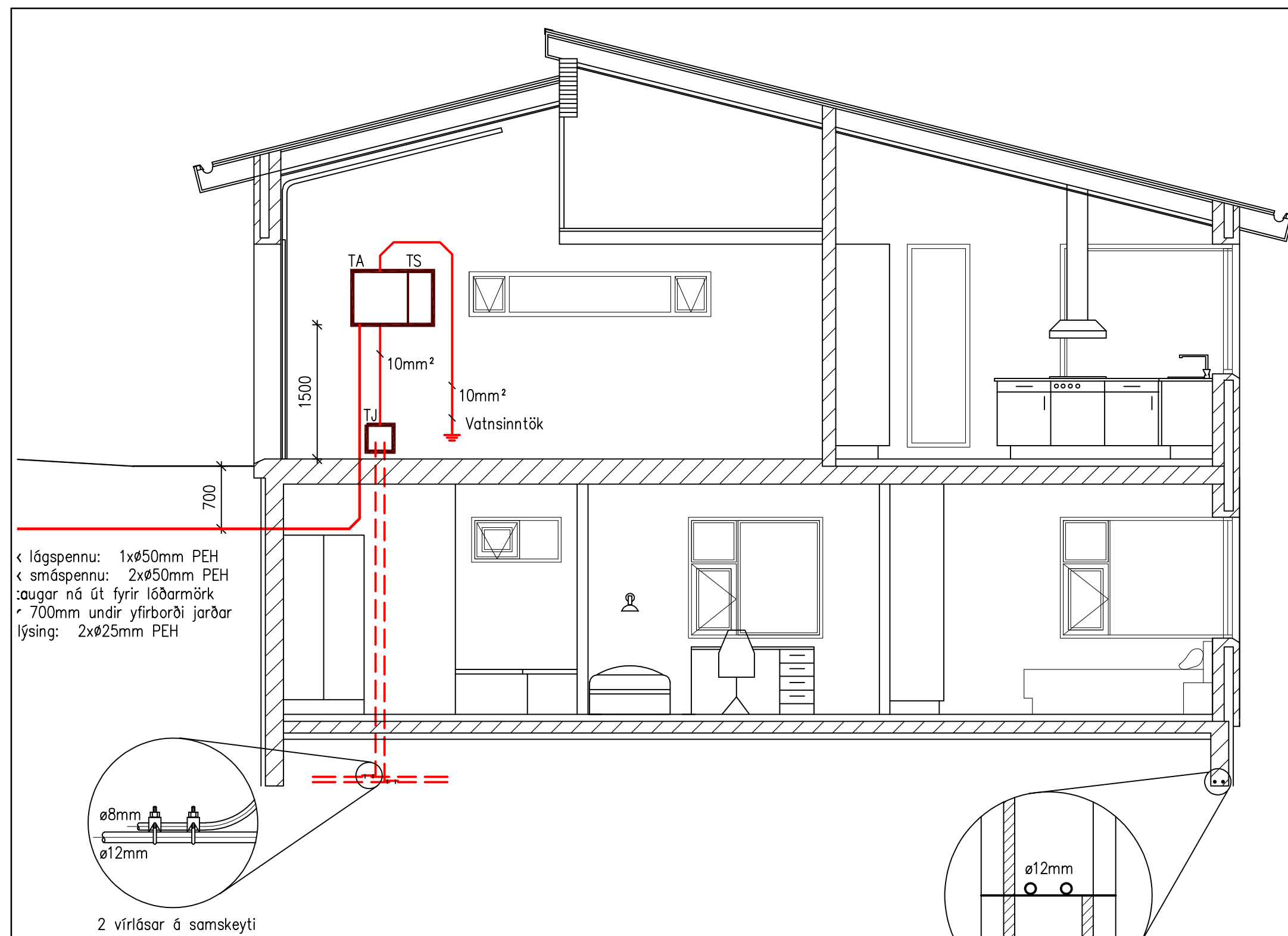
Snið A-A, 1:50
