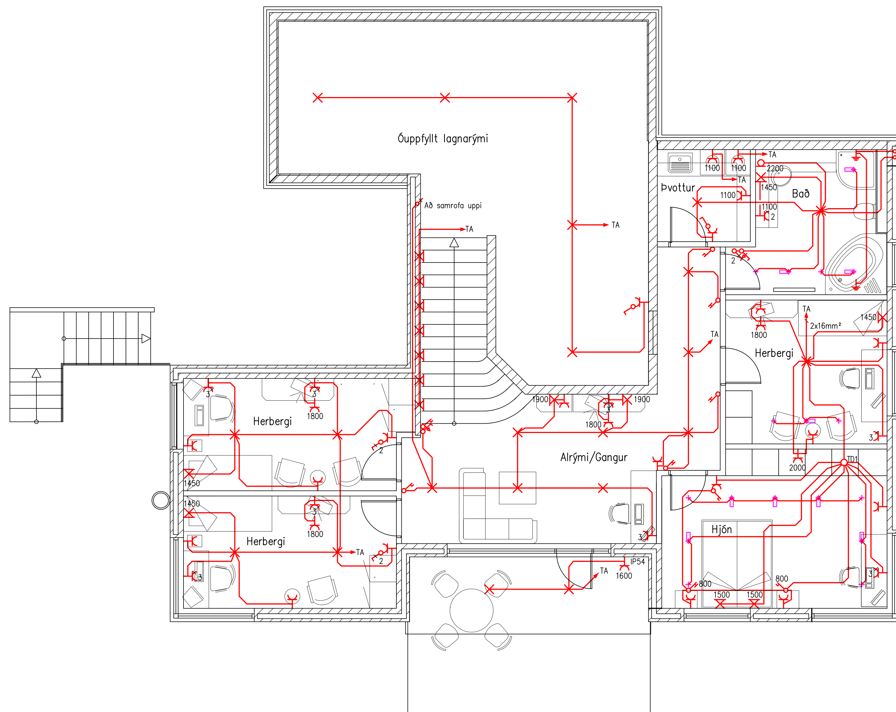
Grunnmynd kjallari, 1:50
