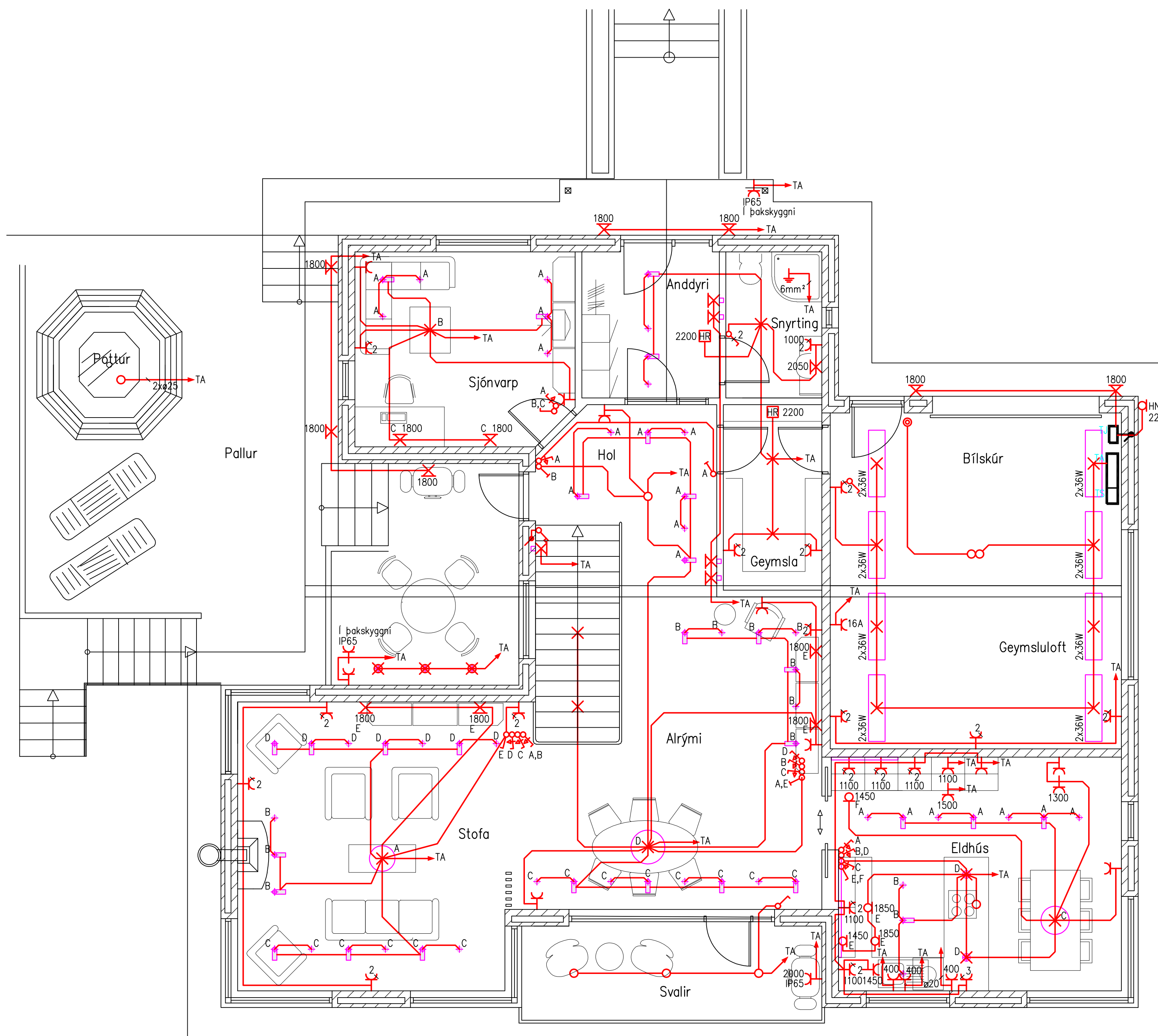
Grunnmynd 1. hæð, 1:50
