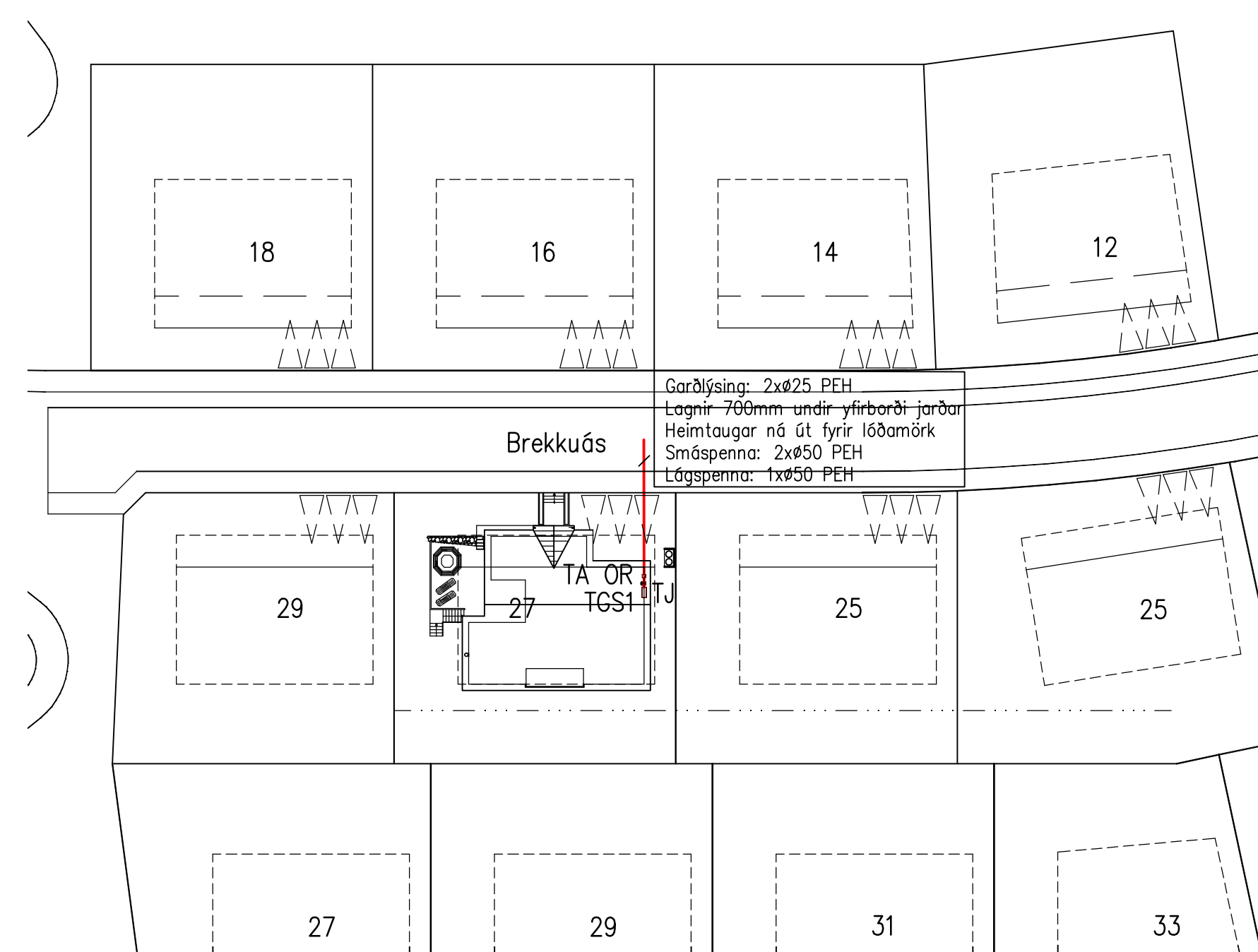
Afstöðumynd, 1:500
