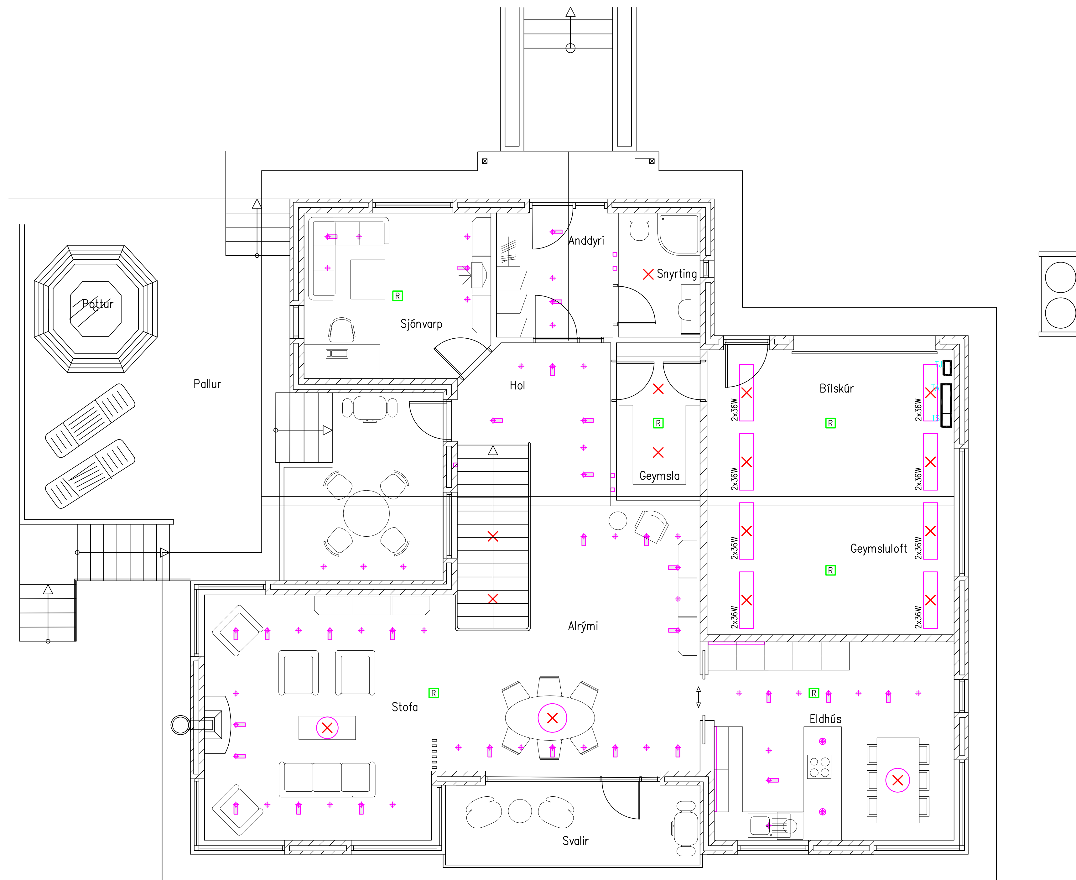
Grunnmynd 1. hæð, 1:50
