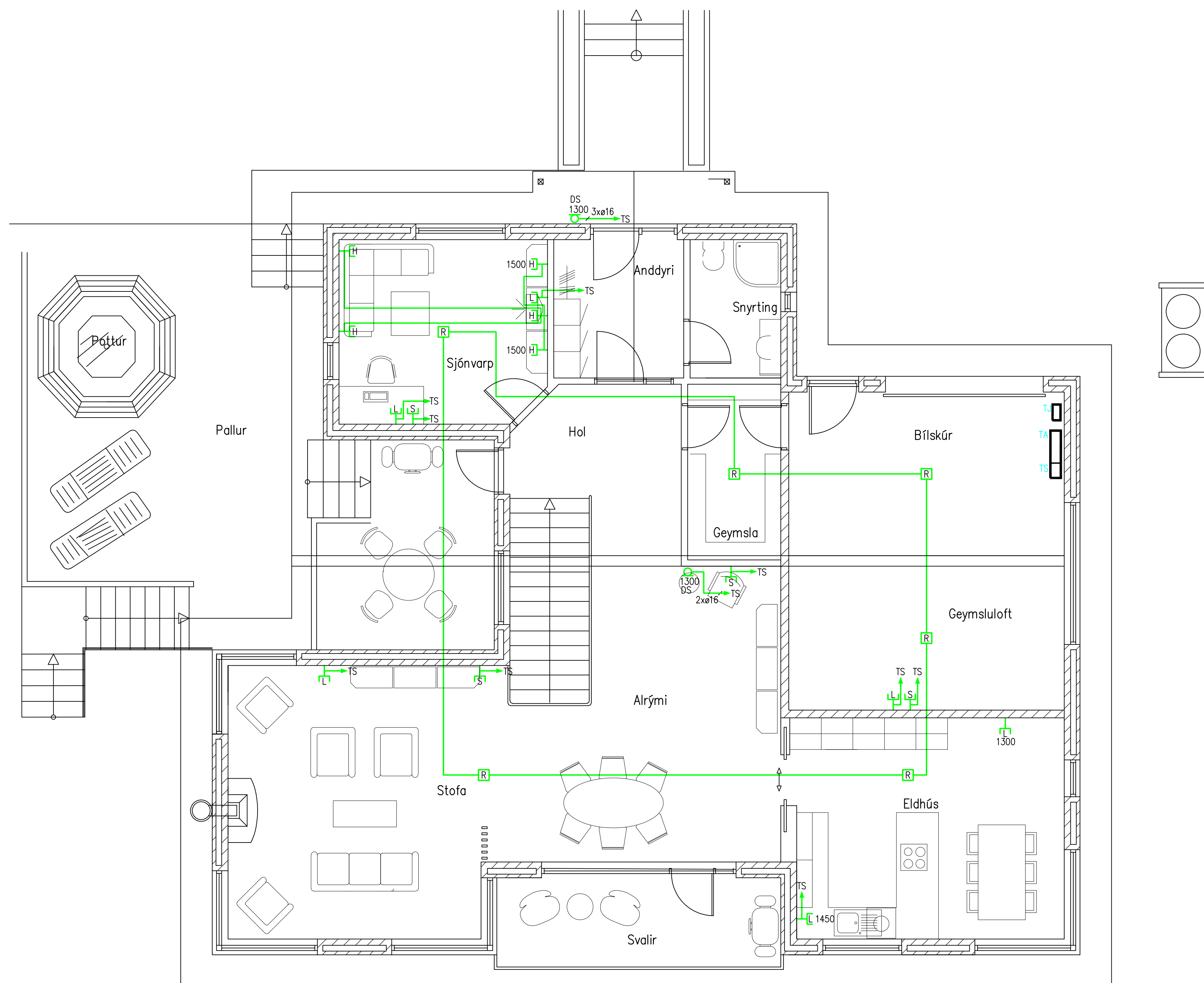
Grunnmynd 1. hæð, 1:50
